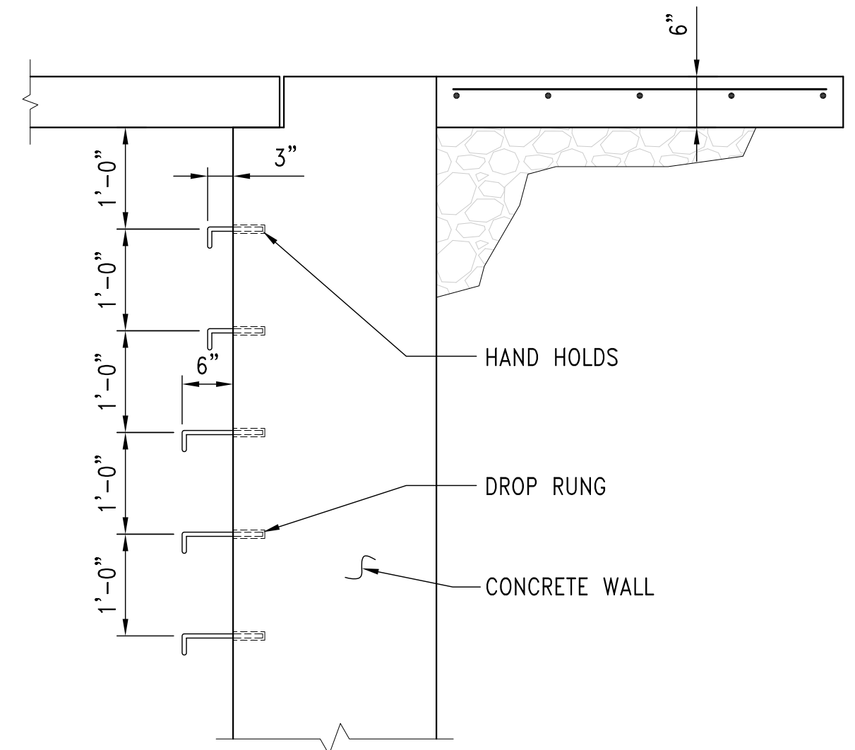
SECTION SCALE: 3/4" = 1'-0"
